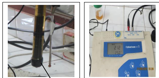
Gambar 1. Rangkaian alat pengukuran potensial ESI
