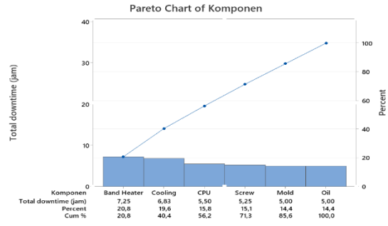
Gambar 1. Diagram Pareto Komponen
