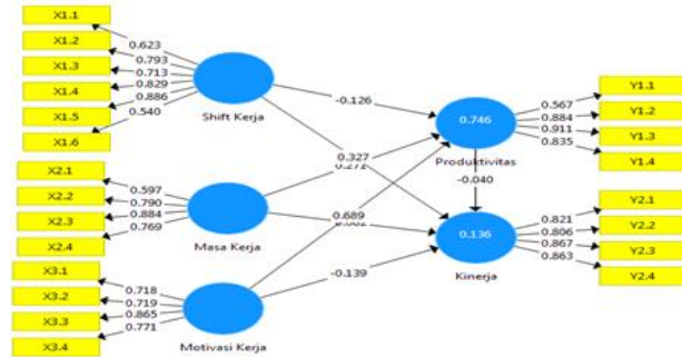
Gambar 1 SEM PLS
